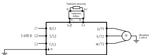
Рис. 3.2г. Подключение силовых клемм
