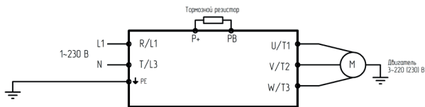
Рис. 3.2б. Подключение силовых клемм
