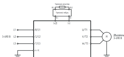
Рис. 3.2.5 Подключение силовых клемм
