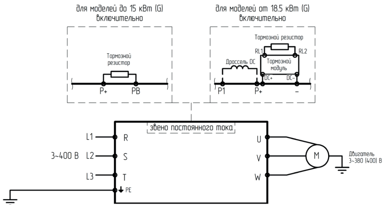
Рис. 2 – Подключение силовых клемм
