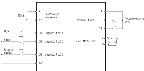
Рис.5а. Подключение клемм управления серии SBIM мощностью до 15 кВт
