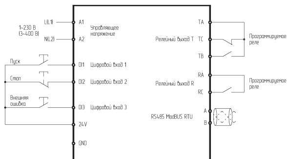
Рис.56. Подключение клемм управления серии SBIM мощностью от 18.5 кВт
